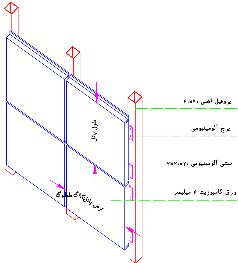
جزئیات نصب ورق کامپوزیت با روش فیکس
